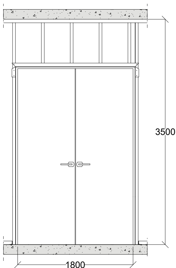
Elevation av dörr
