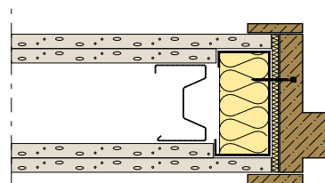
Detalj gyproc GFR 95 som dörrregel
