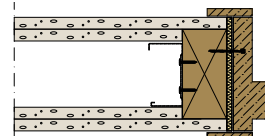
Detalj gyproc ER och träregel
