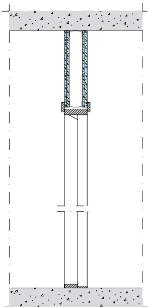
A Sektion 1:20
