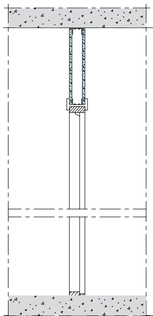
A Sektion 1:20
