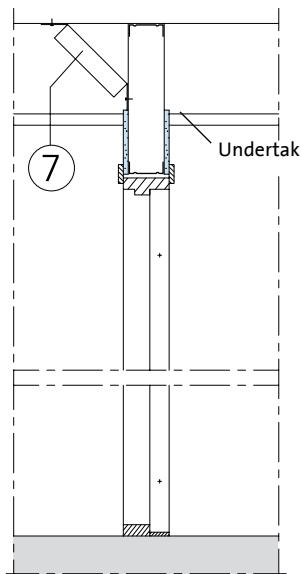
A Sektion 1:20
