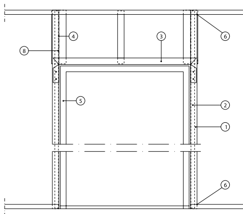
B Elevation 1:20
