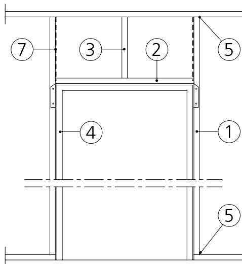
B Elevation 1:20
