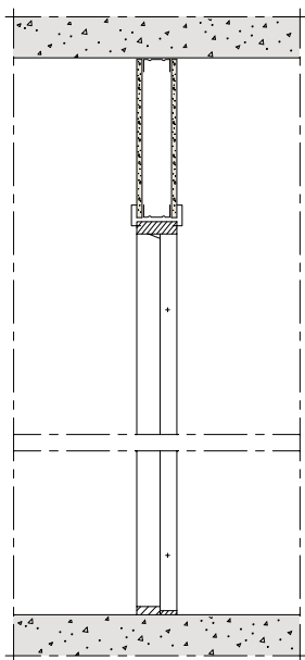
A Sektion 1:20
