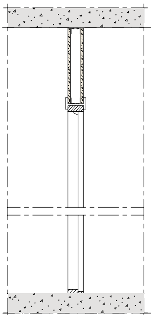
A Sektion 1:20
