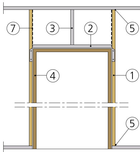
B Elevation 1:20
