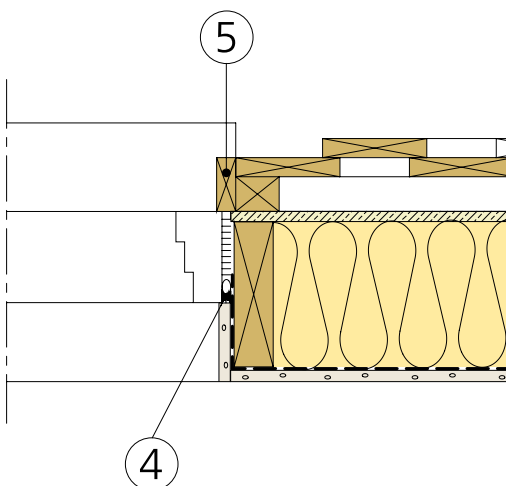
B Horizontalsnitt
