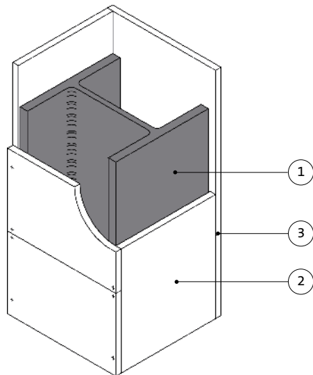
Fyrsidigt inklädd pelare
