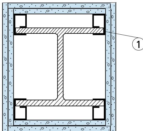
Fig. 1 Fristående pelare
