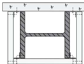
Fyrsidigt inklädd pelare, dubbla skivlag
