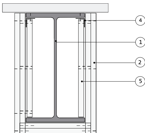
Tresidigt inklädd balk med hörnprofil för brandisolering upp till 120 min, dubbla skivlag
