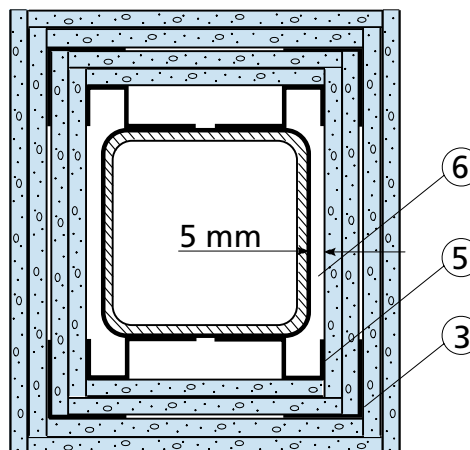
Fig. 3 Fristående pelare
