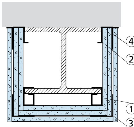
Fig. 2 Balk
